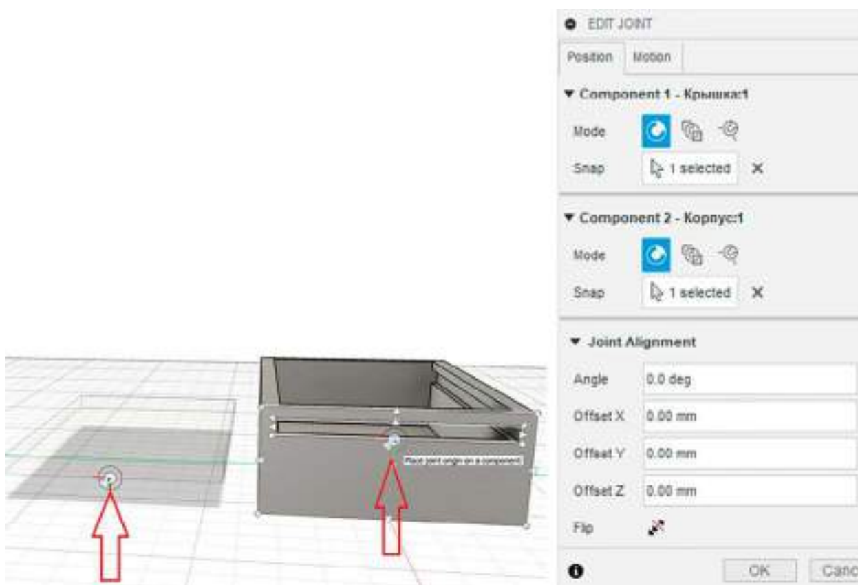
Рис. 17. Точки соединения
